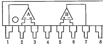
NJM5532L
