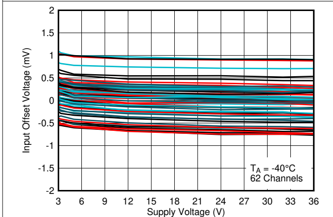
图 6-16. -40°C 下输入失调电压与电源电压之间的关系
