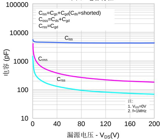
图 5. 电容特性
