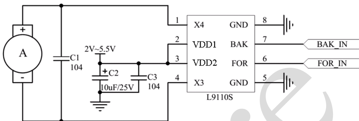
图 4、典型应用图
