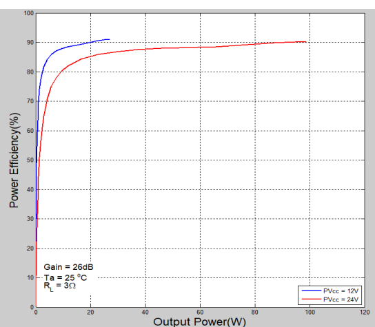
图 9 效率 (PBTL| 3\Omega ) VS 输出功率
