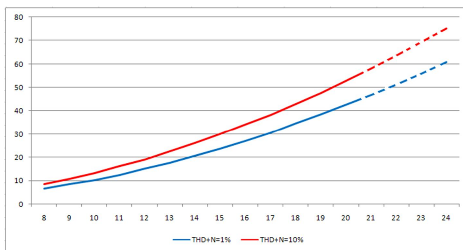
图 3 最大输出功率 (BTL|4Ω) VS 电源电压
