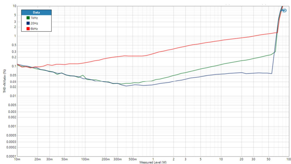
图 15 失真 (PBTL|PVCC=24V|4Ω) VS 输出功率
