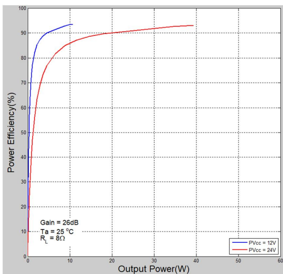
图 6 效率 (BTL| 8\Omega ) VS 输出功率
