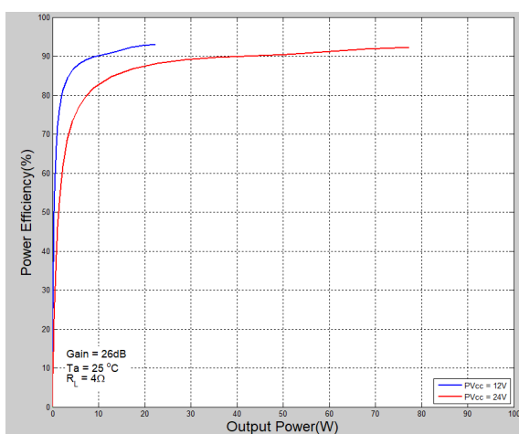
图 8 效率 (PBTL| 4\Omega ) VS 输出功率
