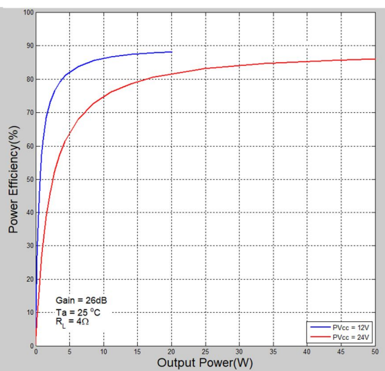
图 7 效率 (BTL| 4\Omega ) VS 输出功率
