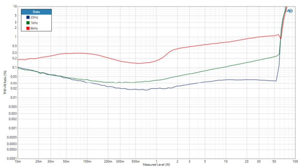
图 14 失真 (BTL|PVCC=24V|4Ω) VS 输出功率
