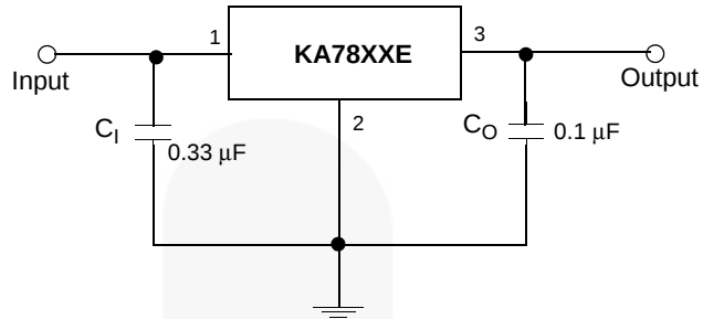
Figure 6. DC Parameters
