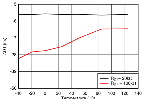
图 6-25. 死区时间匹配与温度之间的关系 ( R_{DT} = 20\text{k}\Omega 和 100\text{k}\Omega )
