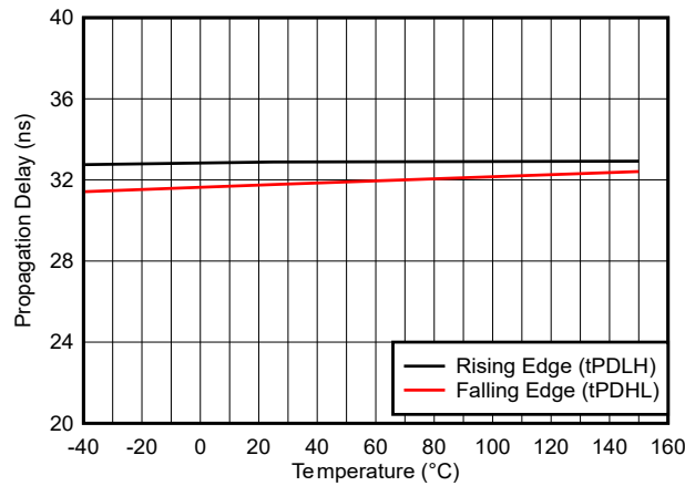
图 6-12. 传播延迟与温度间的关系
