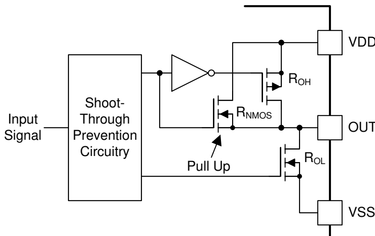
图 8-2. 输出级
