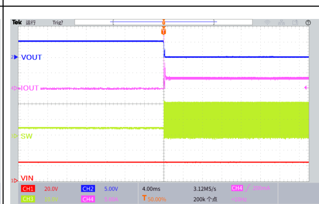
图 29.输出短路波形 ( V_{IN}=24V , V_{OUT}=5.0V )
