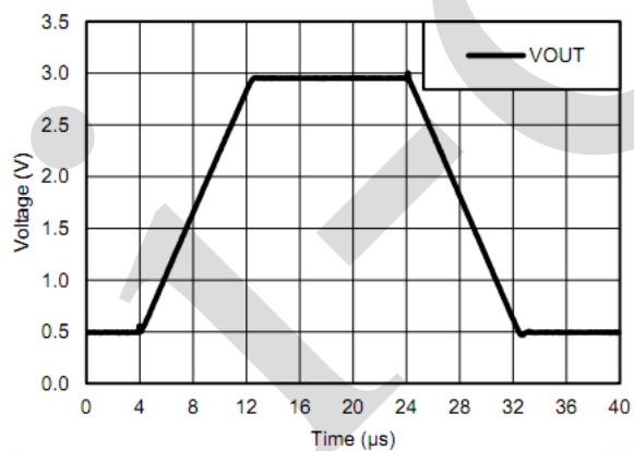
图 5: 电压跟随器大信号响应 (50pF)
