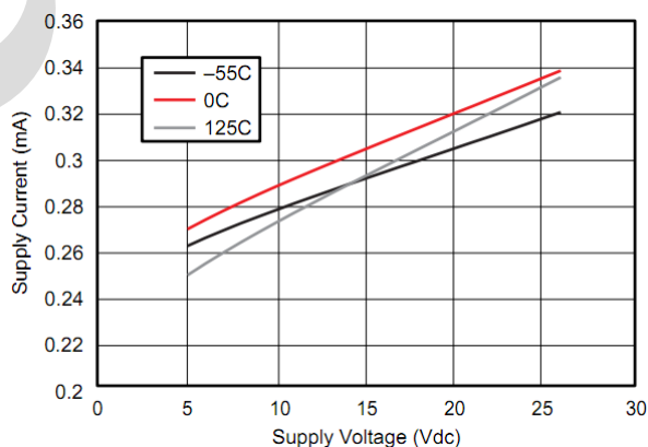
图 2: 工作电流随电源电压变化
