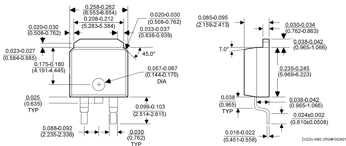
TO-252 PLASTIC PACKAGE (D)
