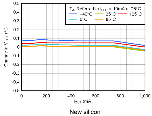
图 5-2. Load Regulation
