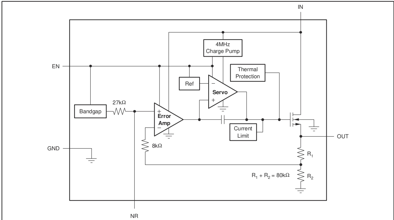
图 6-1. Fixed-Voltage Version
