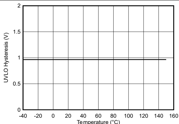
图 5-19. 12V UVLO 迟滞与温度间的关系
