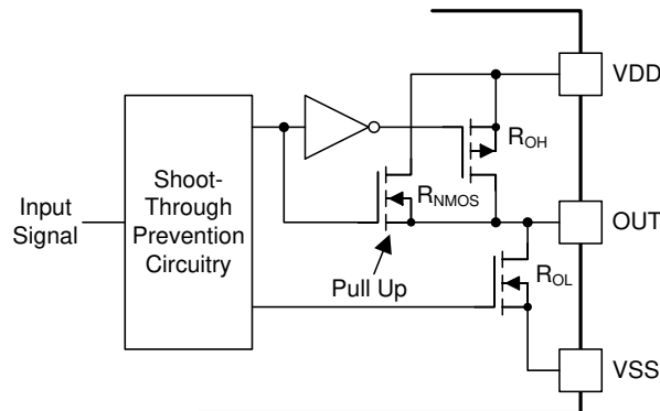
图 7-2. 输出级
