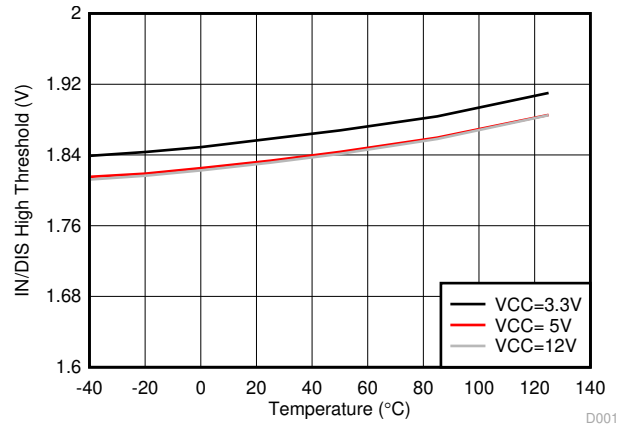
图 5-23. INA/B/EN 高阈值
