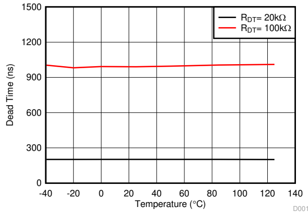
图 5-24. 死区时间与温度间的关系
