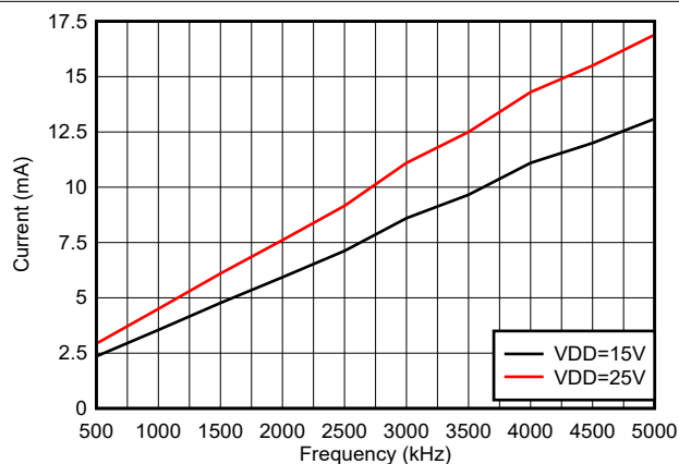
图 5-4. 每通道电流消耗与频率间的关系
