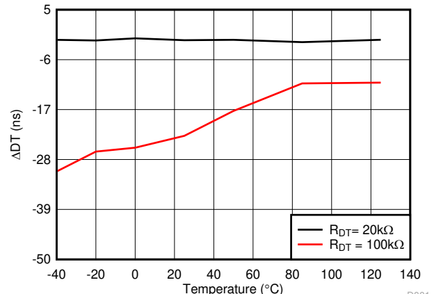
图 5-25. 死区时间匹配与温度间的关系
