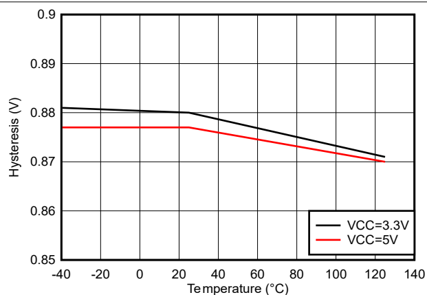
图 5-21. INA/B/EN 迟滞与温度间的关系
