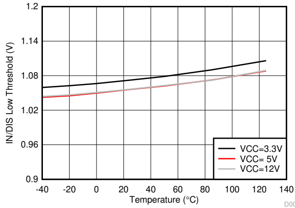
图 5-22. INA/B/EN 低阈值
