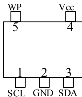
SOT23-5
