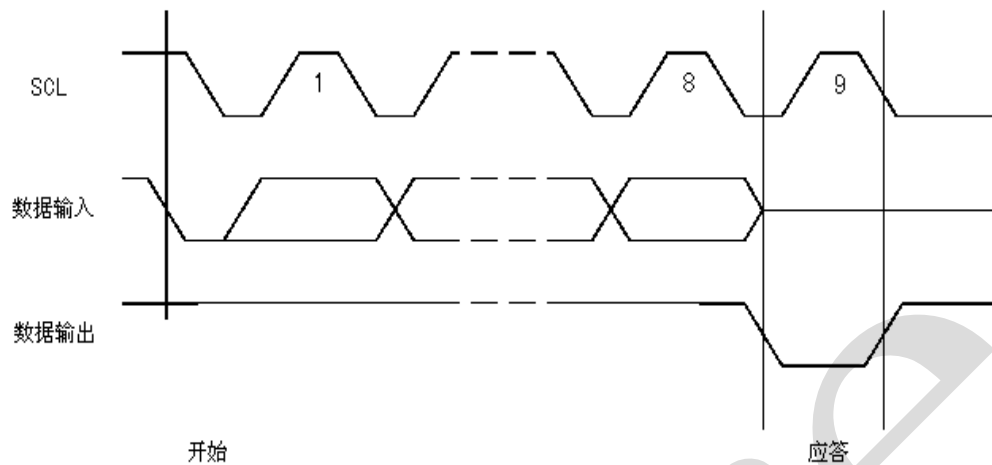
图 7、输出响应
