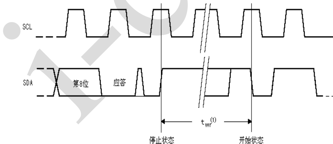
图 6、写周期时序
