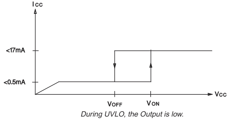
图 6-3. 欠压锁定
