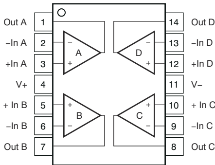
图 4-2. OPA1664：D 和 PW 封装，SOIC-14 和 TSSOP-14 (顶视图)
