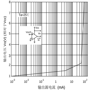
图12 电流限制
