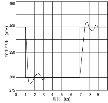
图8 电压跟随器脉冲响应（小信号）
