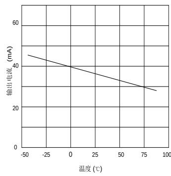
图12 电流限制
