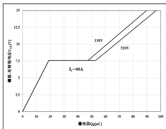
图 18 栅电荷特性
