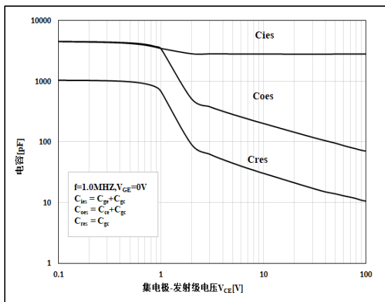
图 5 电容特性
