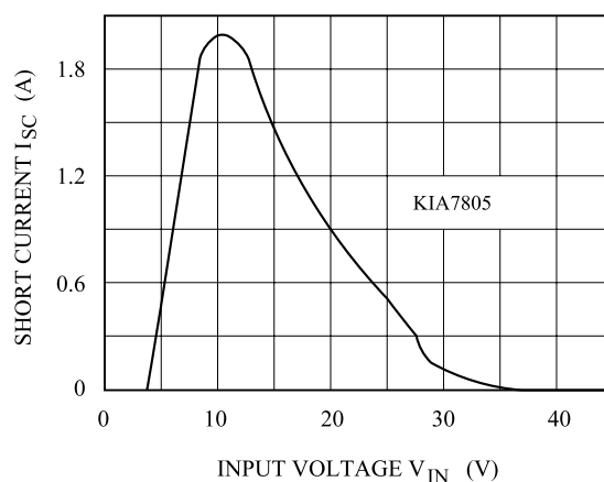
Fig. 7 V_{IN} - I_{SC}
