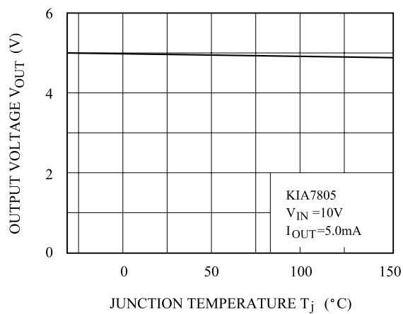
Fig. 5 V_{OUT} - T_j
