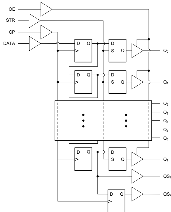
功能框图
