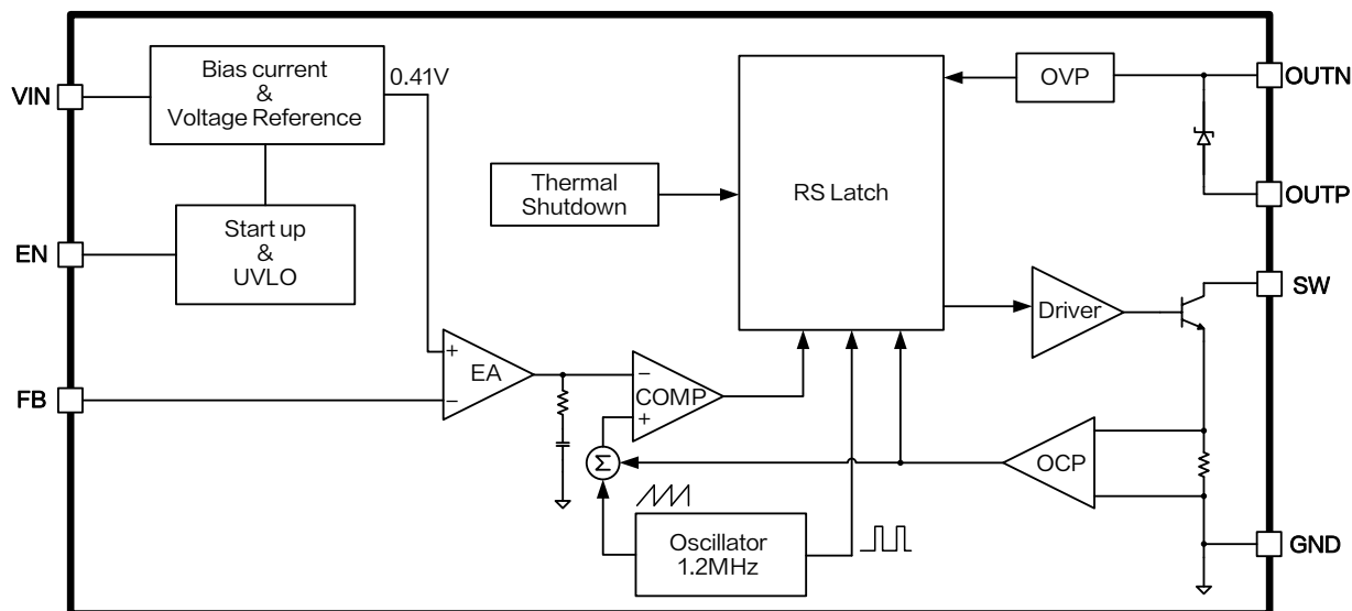
图 3. XL6109 方框图
