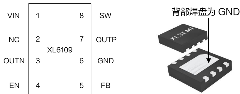
图 2. XL6109 引脚配置
