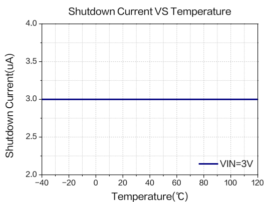
图 10.关机电流温度系数曲线图
