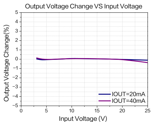
图 8.线性调整率曲线图
