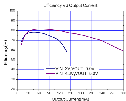
图 4. XL6109 系统参数测量电路及效率曲线图 ( V_{OUT}=5.0V )
