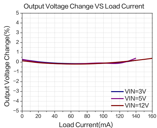
图 9.负载调整率曲线图
