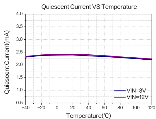
图 11.待机电流温度系数曲线图
