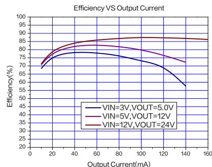
图1.XL6109典型应用示意图和转换效率曲线
