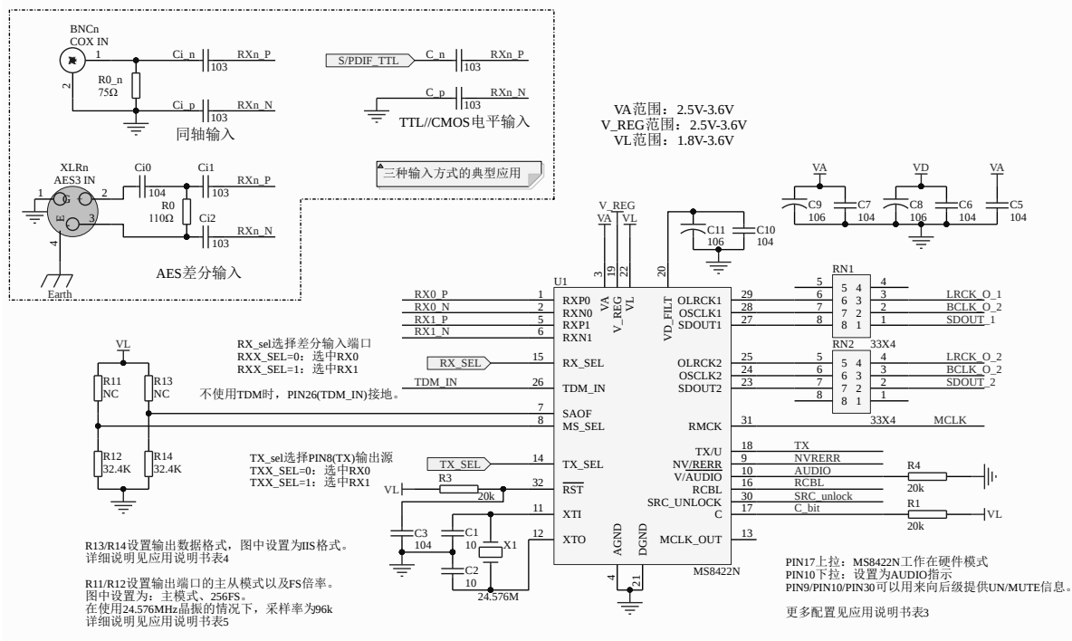
图 8. 硬件模式下典型连接图
