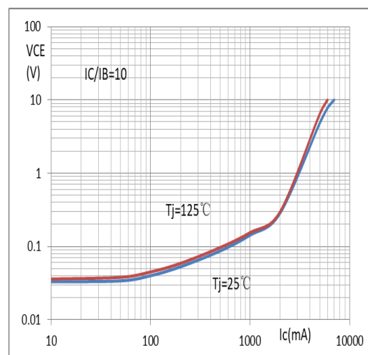
VCE(sat)-Ic
