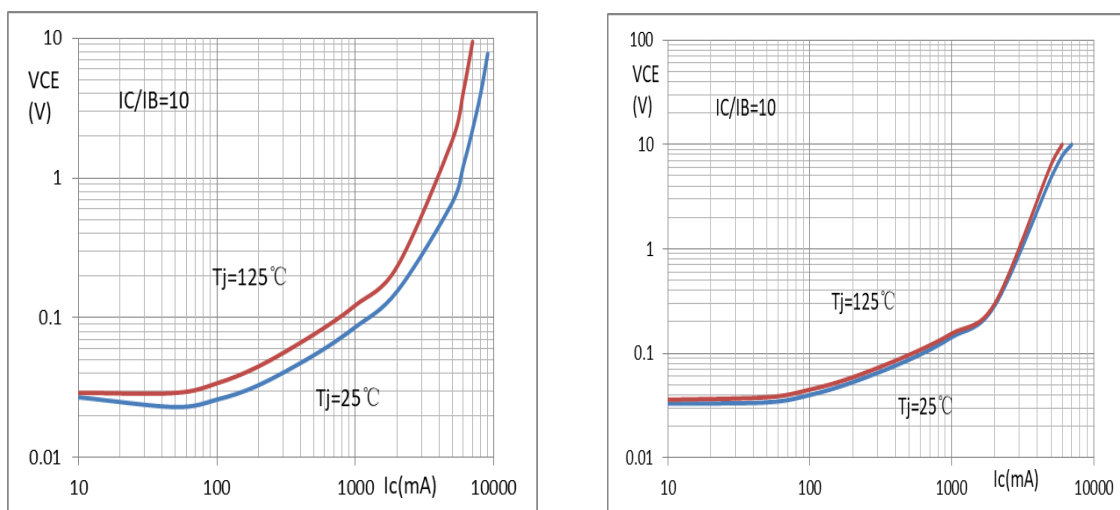
VCE(sat)-Ic
