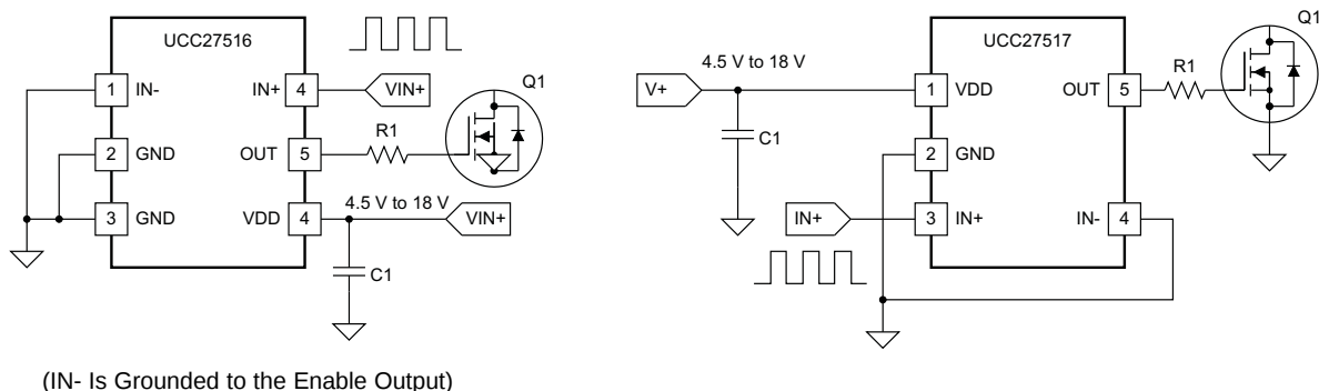
图 24. Using Noninverting Input
