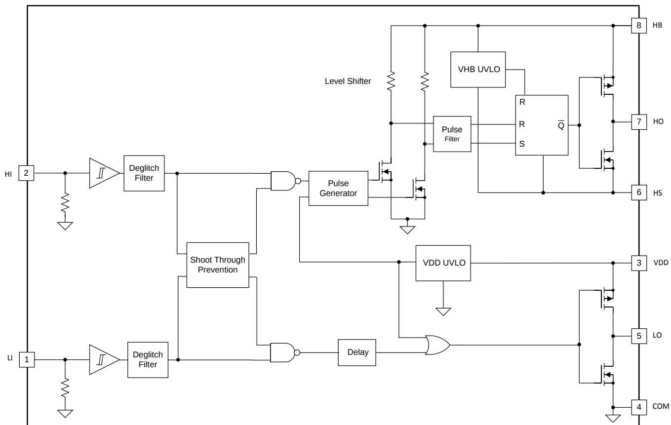
图 29. UCC27712 Block Diagram
