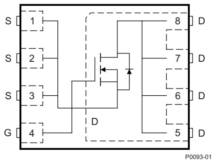
顶视图
