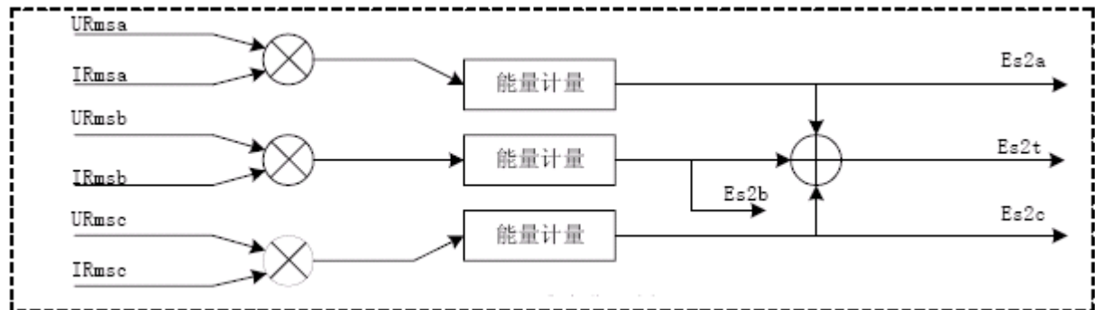
图 2-9-2-2 视在能量测量
