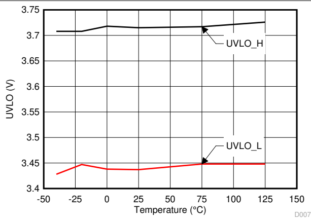
图 5-12. UVLO 阈值
