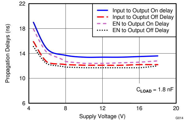
图 6-18. 传播延迟与电源电压间的关系
