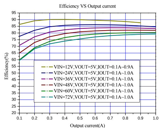
Figure14. VIN=10V~80V, VOUT=5V
