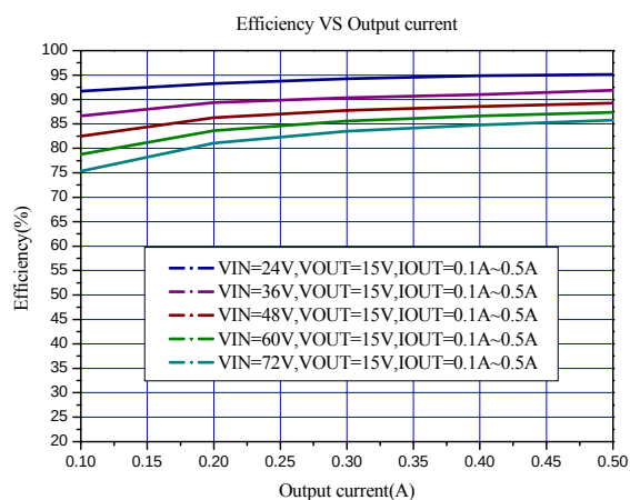
Figure13. VIN=20V~80V, VOUT=15V
