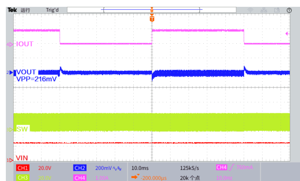
图 33.瞬态负载响应波形 ( V_{IN}=24V , V_{OUT}=5.0V , I_{OUT}=0.1 至 1A )
