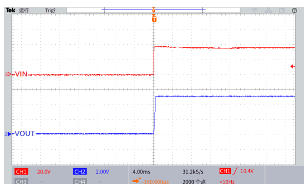
图 26.上电波形图
