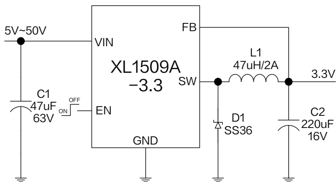
图 8.XL1509A-3.3 系统参数测量电路
