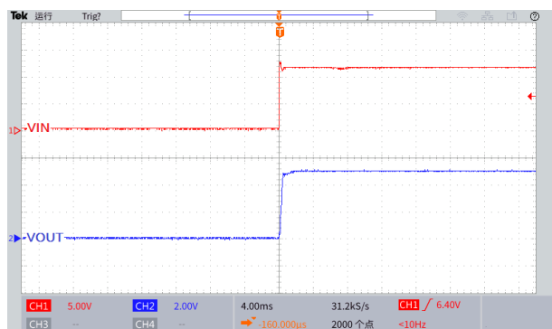
图 24.上电波形图
