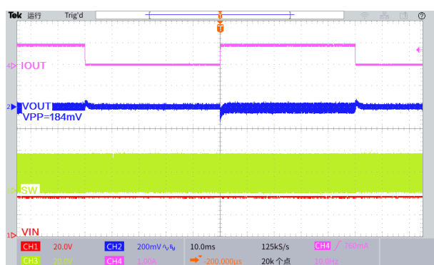
图 34.瞬态负载响应波形 ( V_{IN}=36V , V_{OUT}=5.0V , I_{OUT}=0.1 至 1A )
