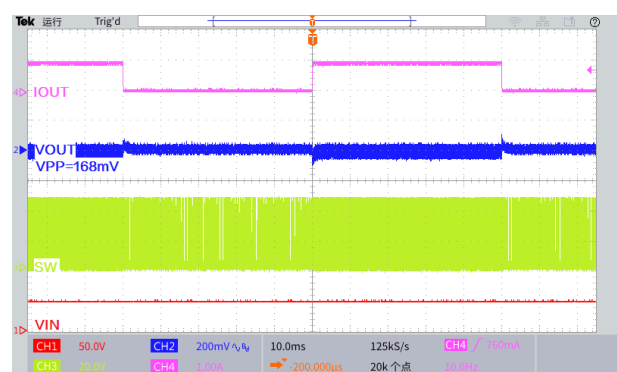
图 35.瞬态负载响应波形 ( V_{IN}=48V , V_{OUT}=5.0V , I_{OUT}=0.1 至 1A )
