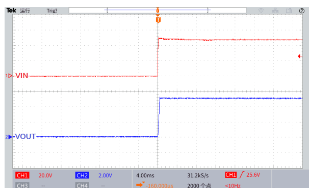
图 27.上电波形图
