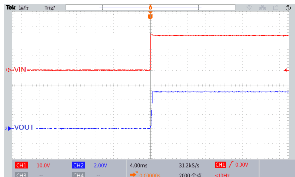
图 25.上电波形图
