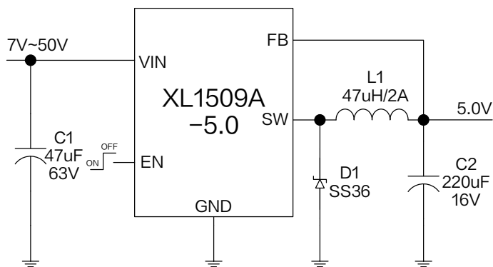
图 10.XL1509A-5.0 系统参数测量电路
