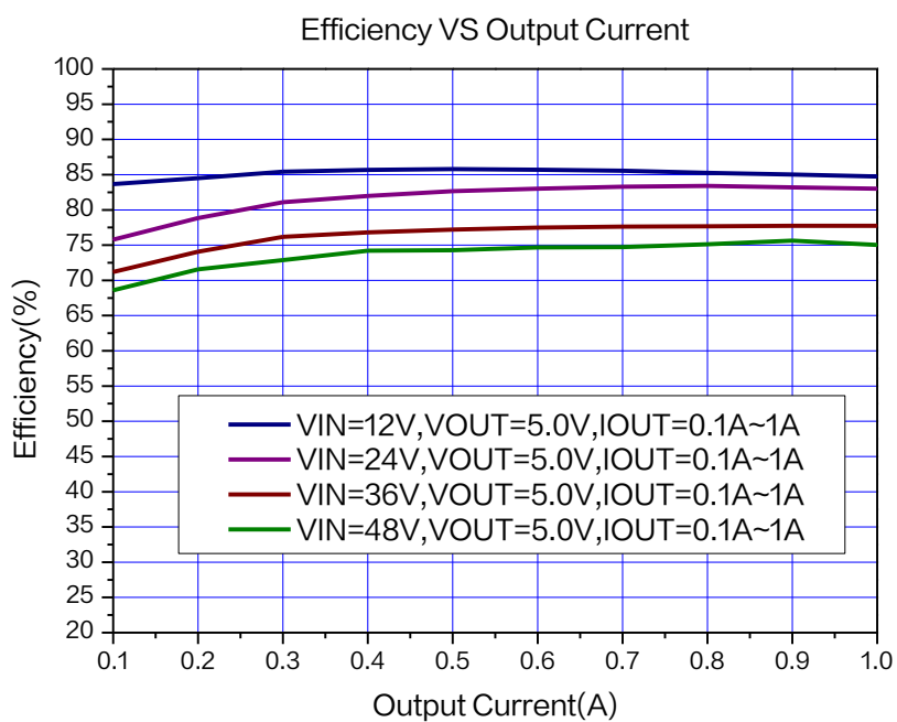
图 11. XL1509A-5.0 系统效率曲线
