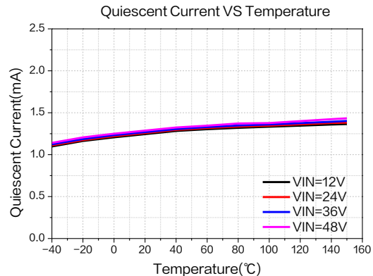
图 19.静态电流温度系数曲线图
