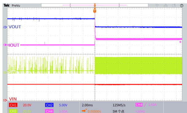
图 30.输出短路波形 ( V_{IN}=36V , V_{OUT}=5.0V )
