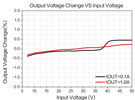
图 14.线性调整率曲线图
