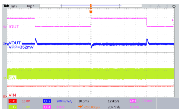
图 32.瞬态负载响应波形 ( V_{IN}=12V , V_{OUT}=5.0V , I_{OUT}=0.1 至 1A )
