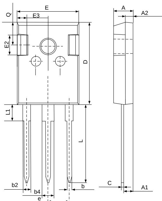
TO-247-3L
