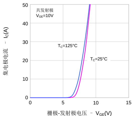
图4. 传输特性
